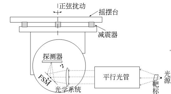
图 13 成像系统原理示意图
