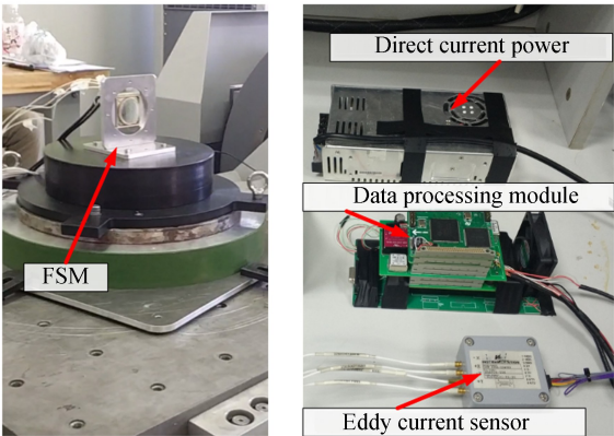
图 9 快速反射镜硬件实验平台
