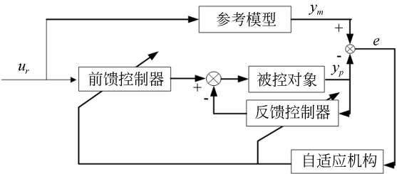
图 2 MRAC 控制系统结构框图
