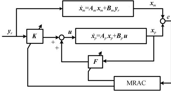
图3 用状态方程描述的MRAC系统框图
