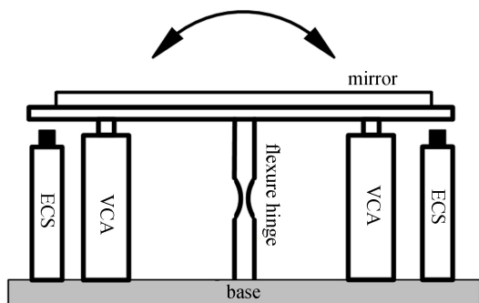
图 4 快速反射镜结构示意图
