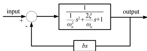
图 6 带速率反馈的二阶系统示意图
