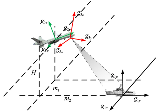
图1 航空成像系统几何关系图
